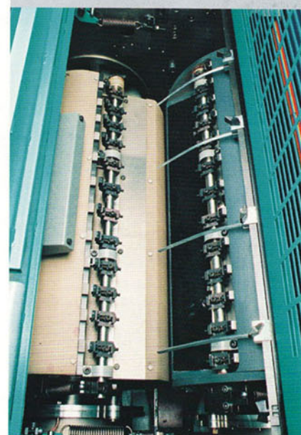
Механизмы захватов передоточных цилиндров
