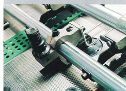
Электромеханический датчик двойного листа
